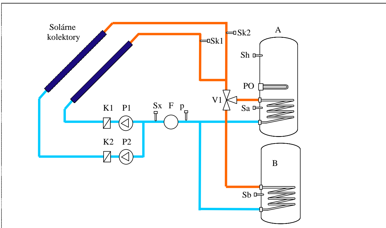
Obr.4 Hydraulická schéma regulovanej sústavy s dvoma kolektorovými poliemi: A, B - výmenníky, Sk1, Sk2, Sa, Sb, Sx, Sh - snímače teploty, p - snímač tlaku, F - snímač prietoku, PO - pomocný ohrev, V1 - prepínací ventil, P1,P2 - čerpadlá, K1,K2 - spätné klapky
